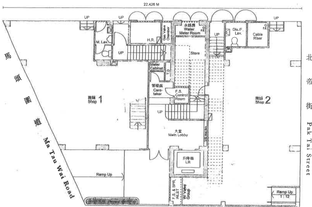
地下平面圖 Ground Floor Plan
